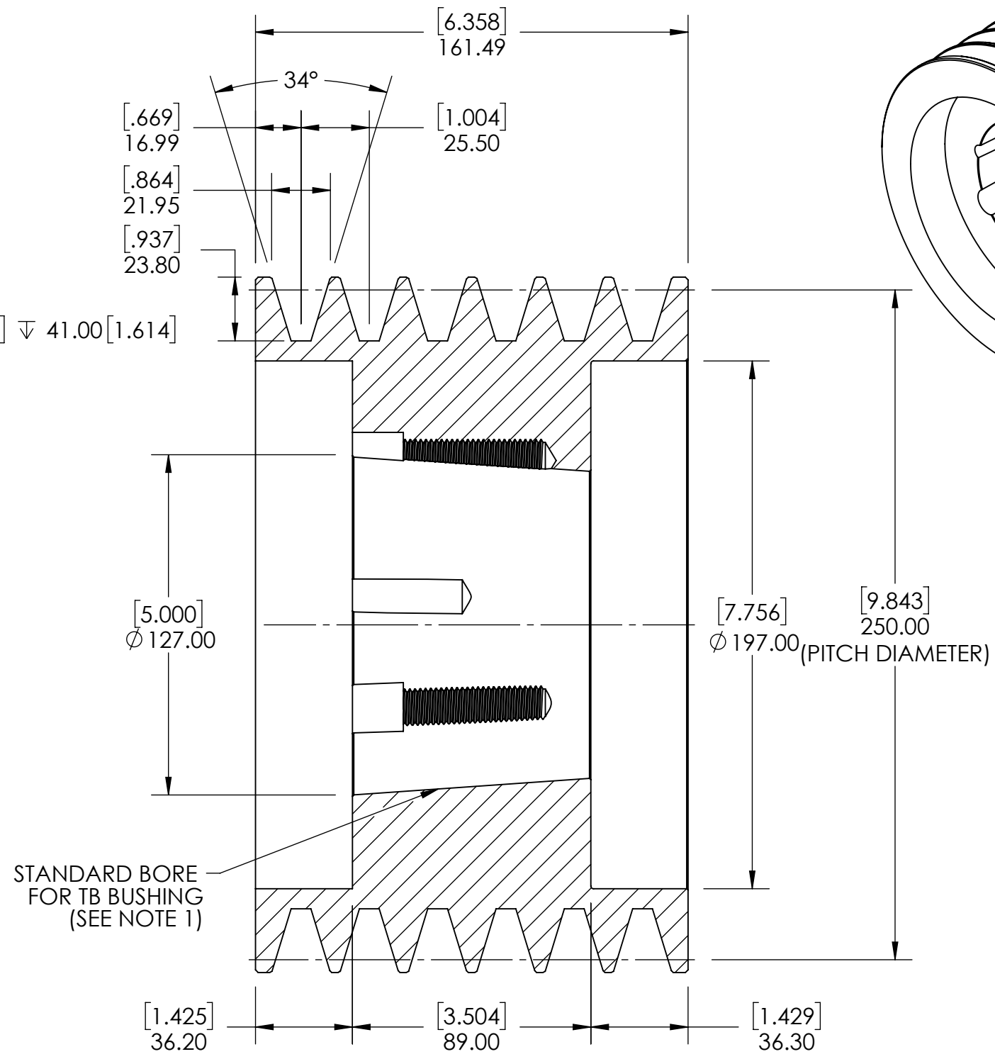
SECTION A-A
