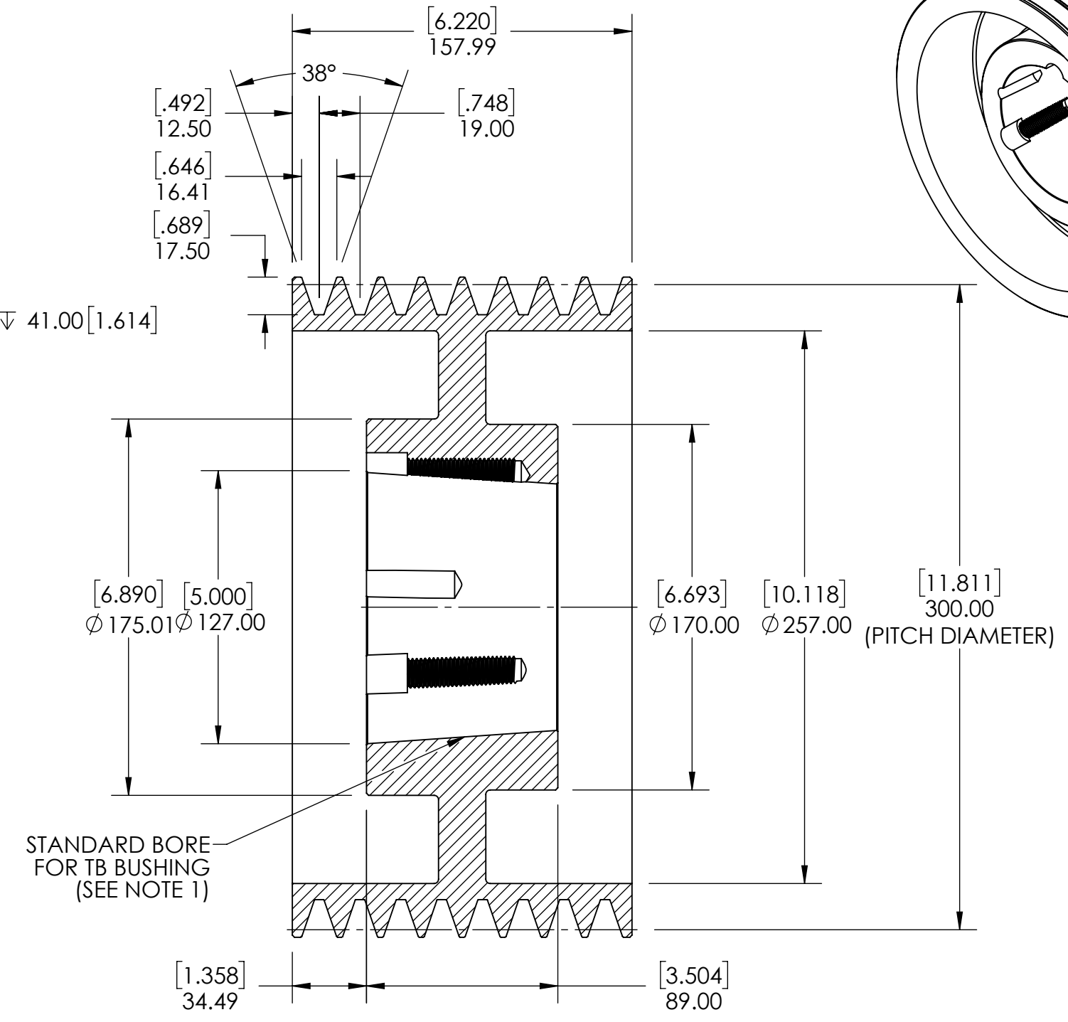
SECTION A-A
