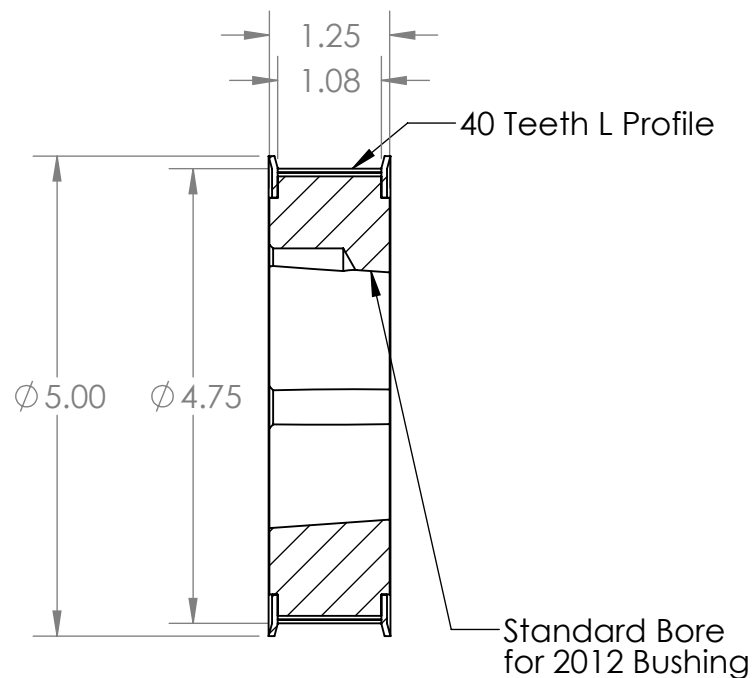
SECTION A-A
