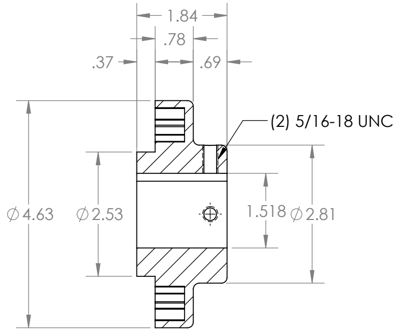
SECTION A-A
