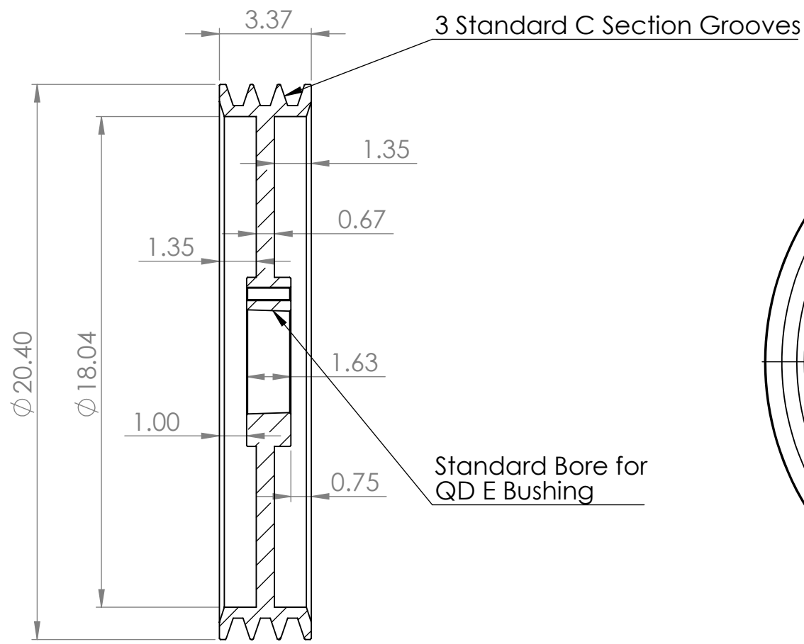
SECTION A-A
