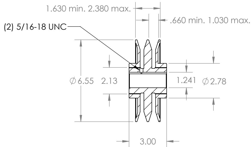
SECTION A-A
