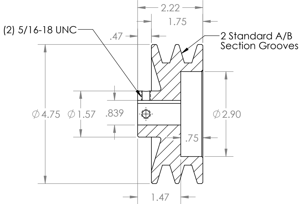
SECTION A-A
