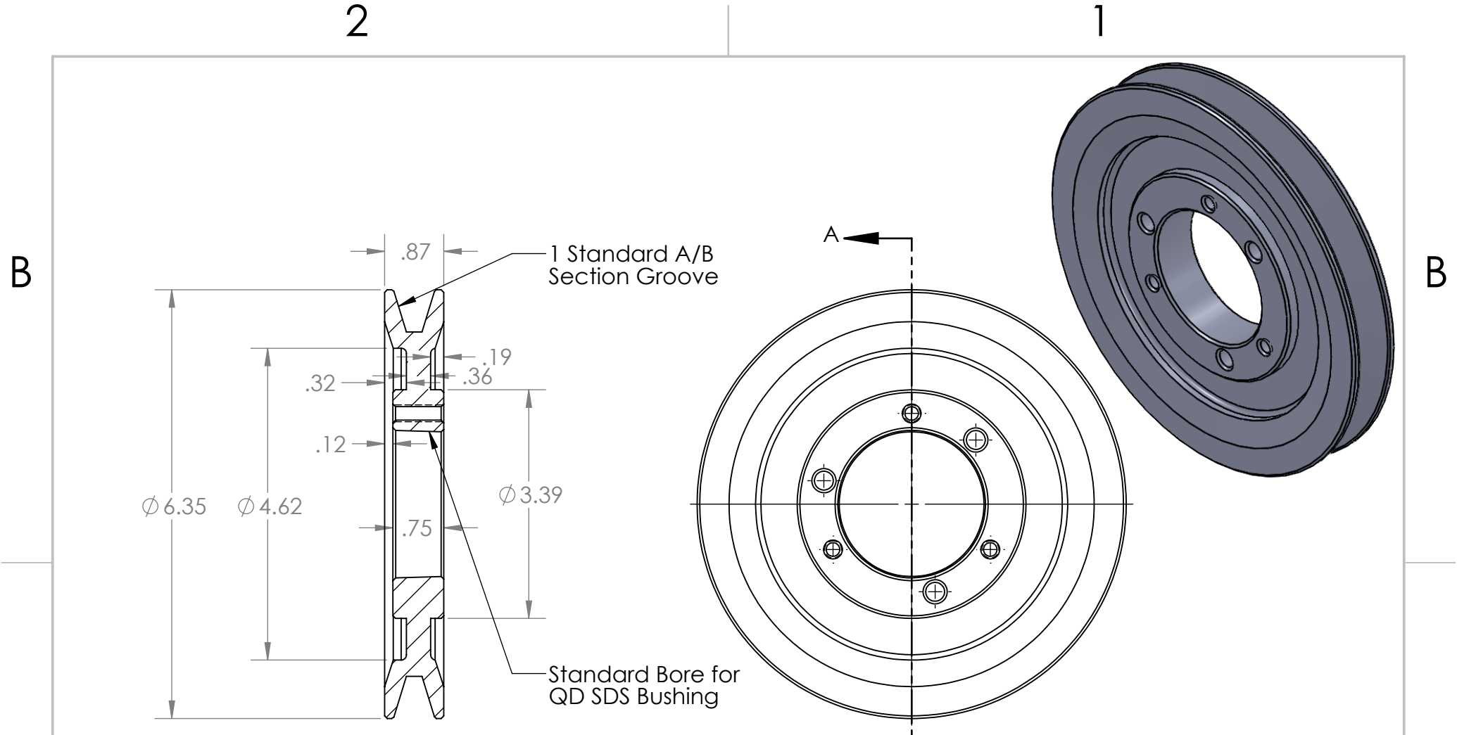
SECTION A-A
