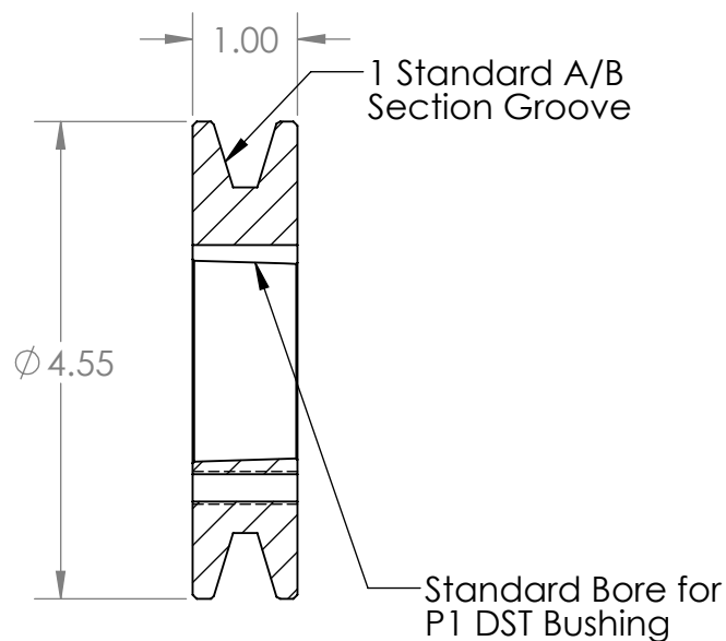
SECTION A-A
