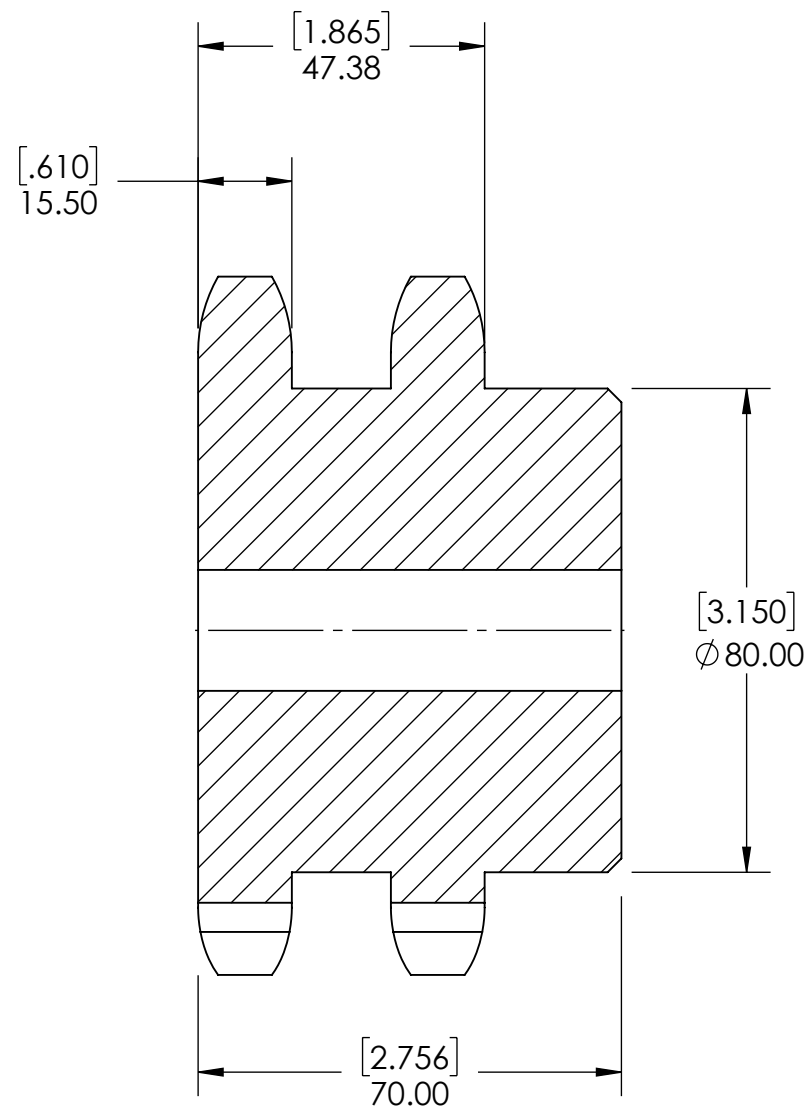
SECTION A-A
