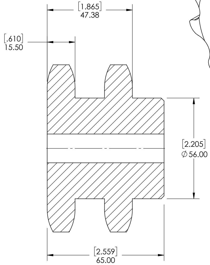
SECTION A-A
