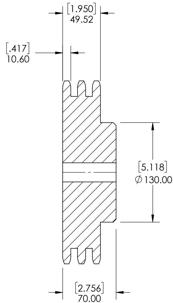
SECTION A-A
