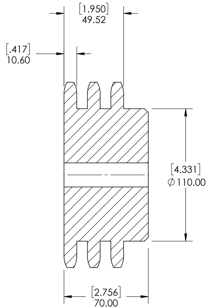
SECTION A-A
