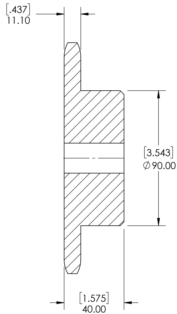
SECTION A-A
