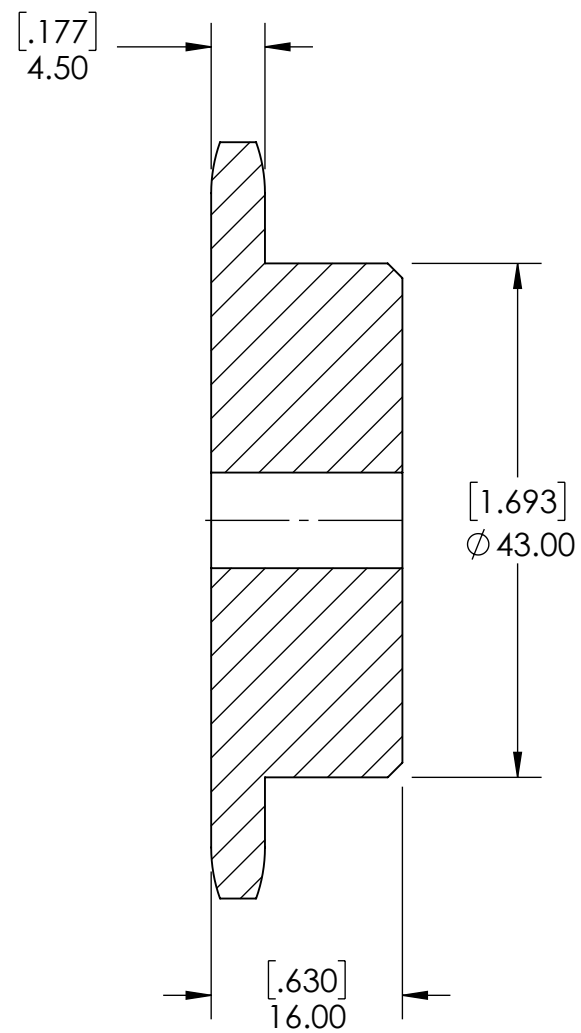
SECTION A-A
