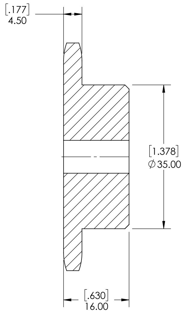
SECTION A-A
