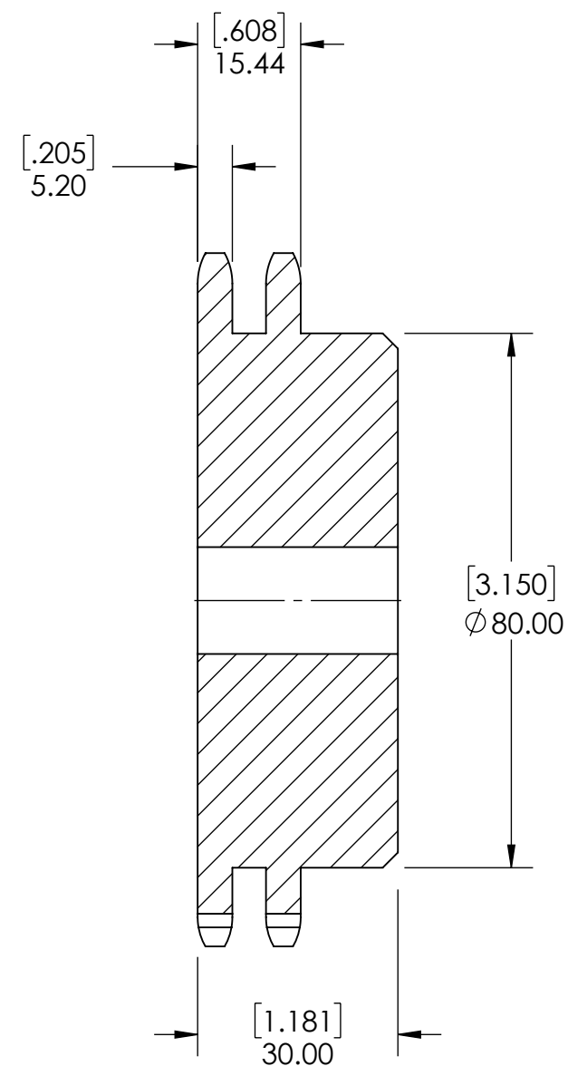
SECTION A-A
